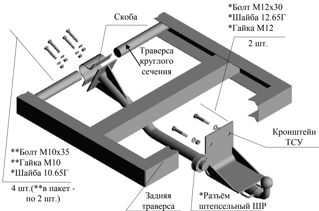
Примечание: детали, помеченные * входят в пакет комплектующих Рис.1 Тягово-сцепное устройство ТСУ 2705
